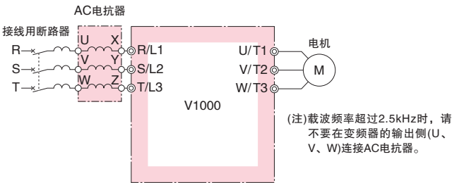
接线图
