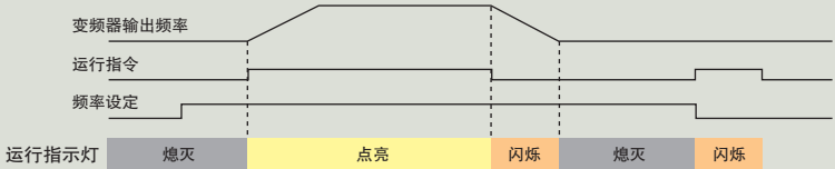
运行指示灯和变频器的动作关系
