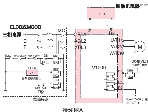
接线图A
