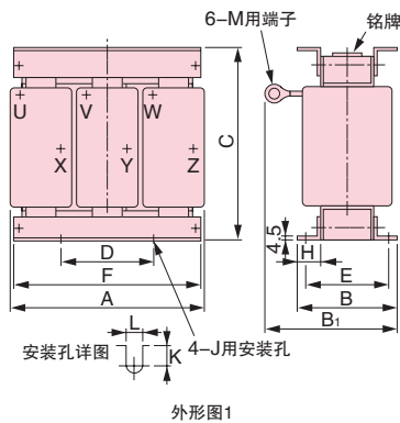
外形尺寸 mm
