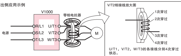
接线图a
