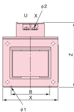
外形图 2
