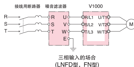
schaffner EMC(株)制 噪音滤波器
