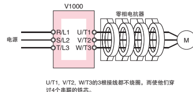
接线图b
