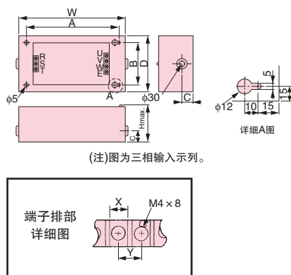
简易型噪音滤波器(带盒) 外形尺寸mm
