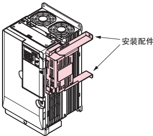
单元(PS-V10M)和安装配件都安装时
