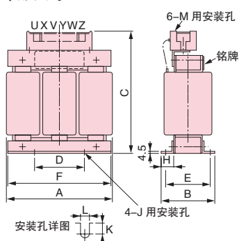
外形尺寸 mm
