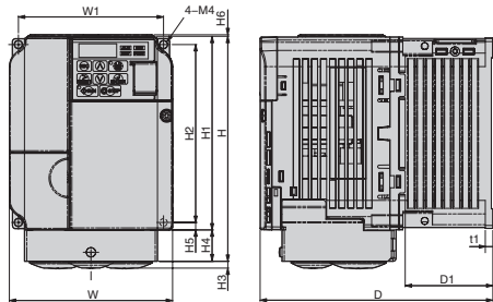
外形图 2
