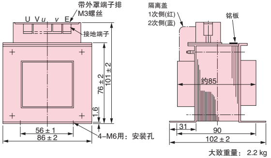
外形尺寸 mm
