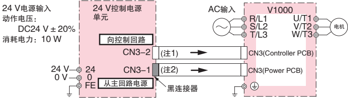
连接图
