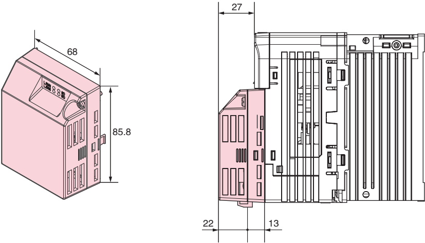
CIMR-VB2A0004 示例
