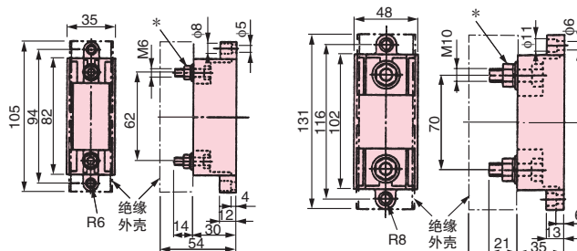
外形图1
