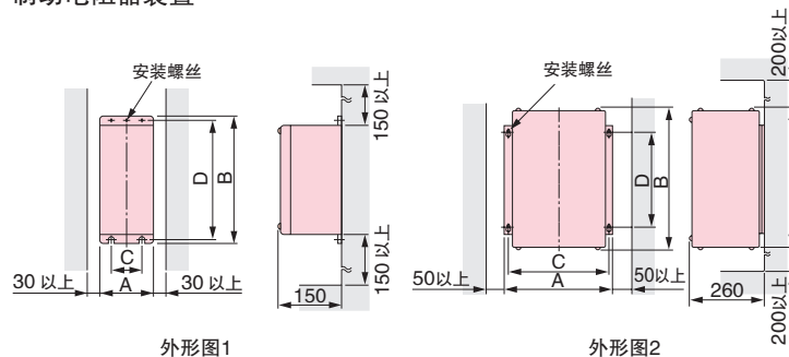
外形图1
