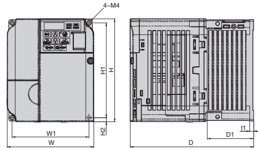
外形图 3
