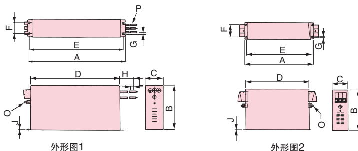
schaffnerEMC(株)制噪音滤波器 外形尺寸mm
