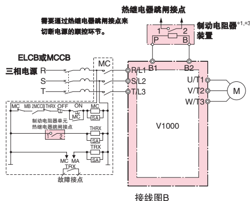
接线图B
