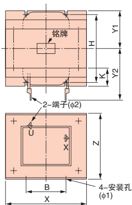
外形图2
