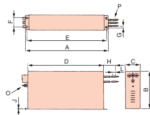
外形图1
