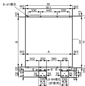
面板加工图4
