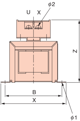
外形图1
