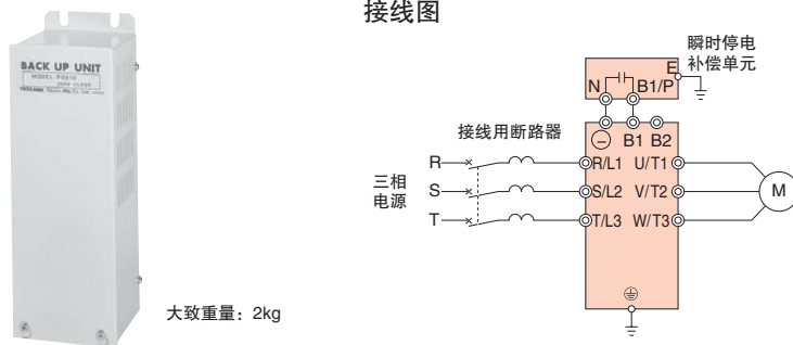
接线图
