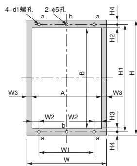
面板加工图1
