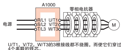
接线图b
