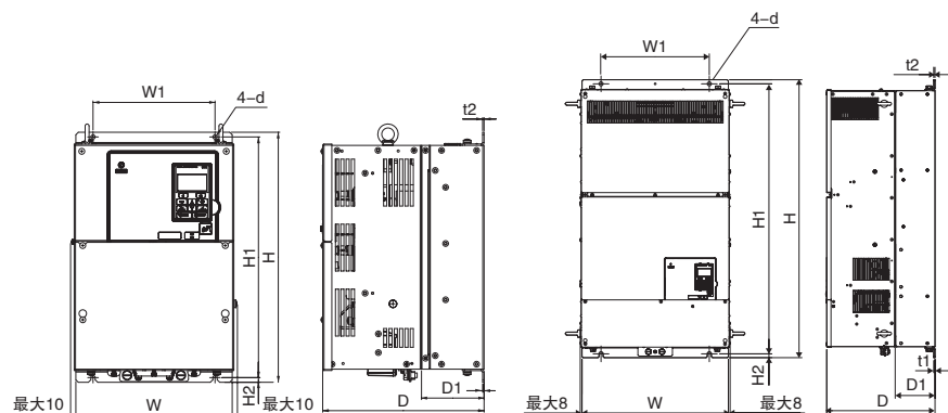
外形图1
