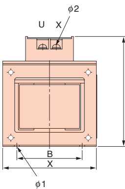
外形图2
