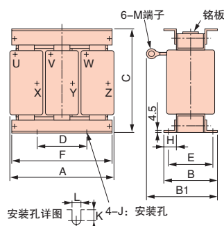
外形图1
