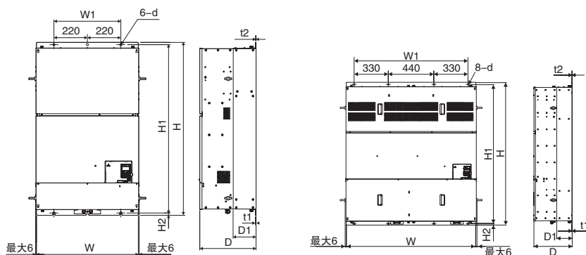
外形图3
