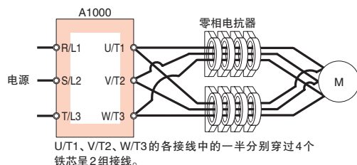
接线图c
