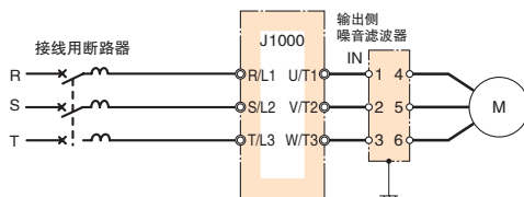
连接图
