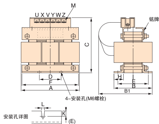
外形图 2
