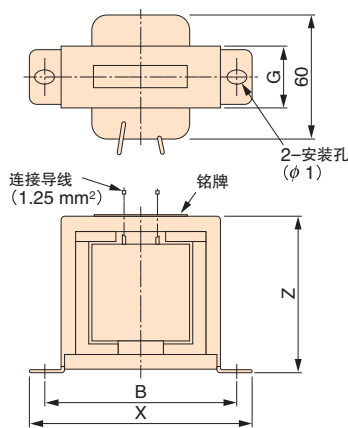
外形图 1
