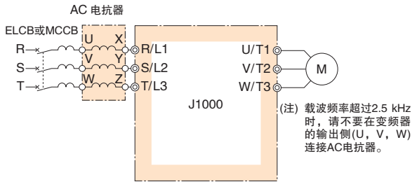
连接图
