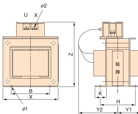
外形图2
