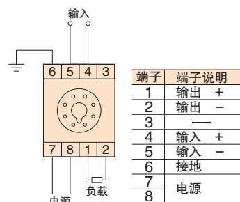
连接图
