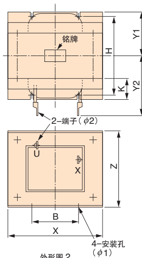
外形图 2
