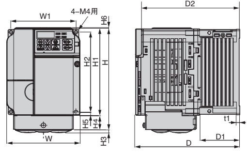
外形图 2
