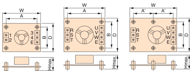
外形图1(单相输入)
