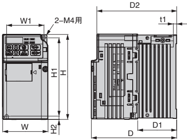
外形图1
