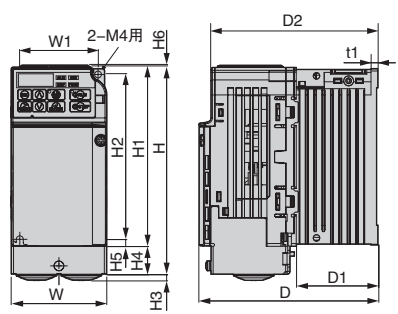
外形图 1
