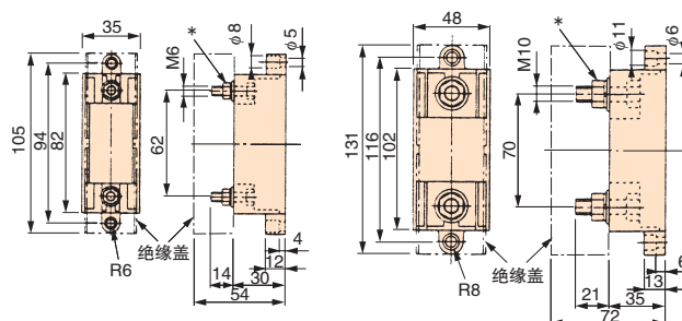
外形图1
